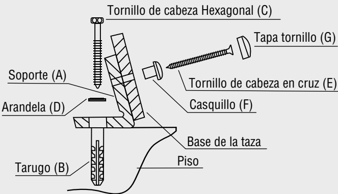
COMPONENTES KIT DE ANCLAJE OCULTO
